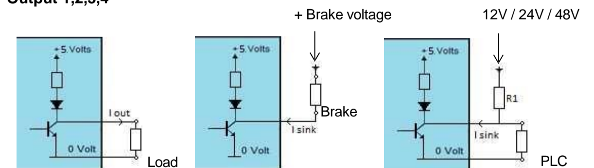
Output 1,2,3,4
