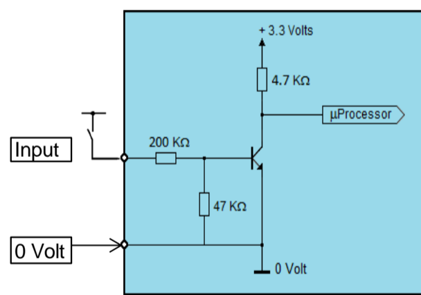
Inputs 1, 2, 3, 4
