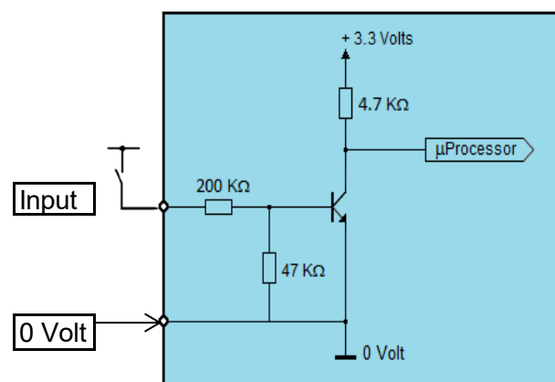
Inputs 1, 2, 3, 4
