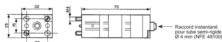
81 502 322 - 81 505 321
