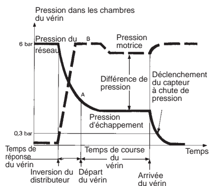
Evolution des pressions dans les chambres d'un vérin à double effet
