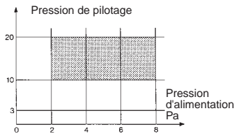
Sortie positive
