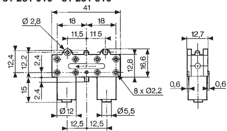
81 281 010 - 81 281 510
