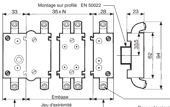
Raccord instantané pour tube semi-rigide Ø 4 mm (NFE 49100)
